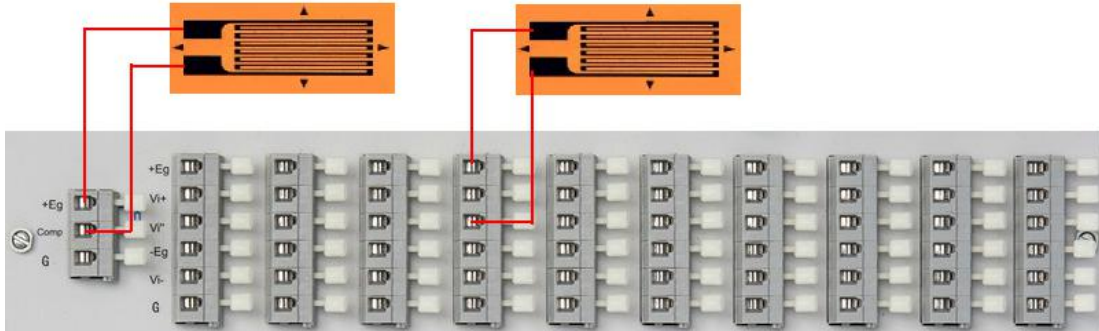
面板设置，根据所接通道桥路设置
