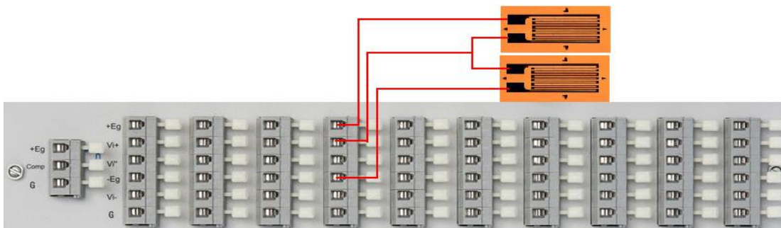
面板设置，根据所接通道桥路设置。
