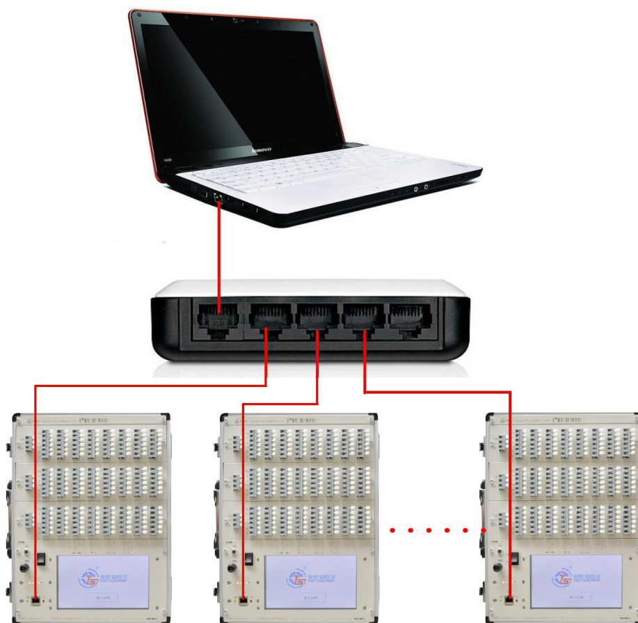
多台仪器网络 HUB 扩展连接图
