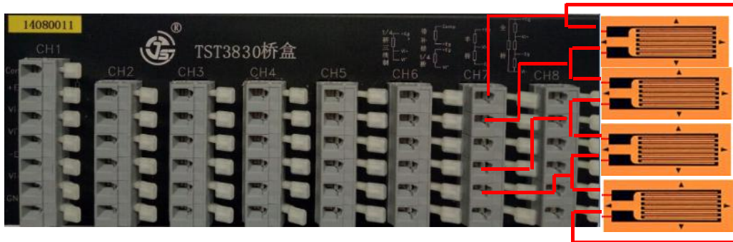
(4) 全桥
