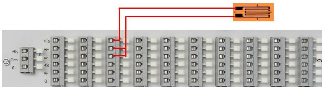
(1) 1/4 桥三线制
