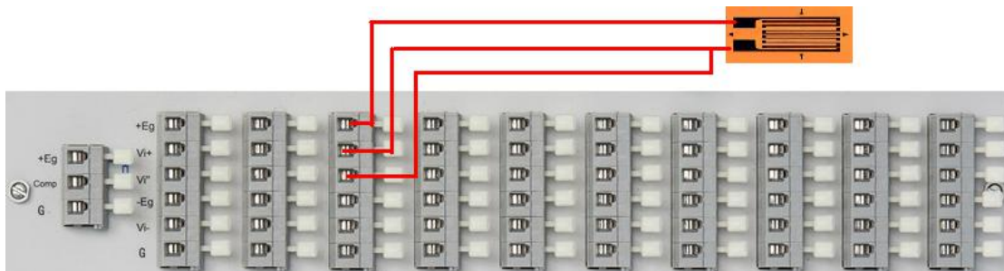
(1) 1/4 桥三线制
