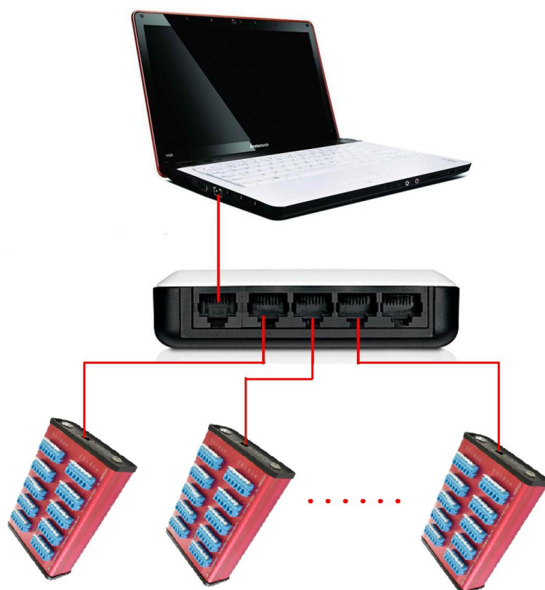
多台仪器网络 HUB 扩展连接图
