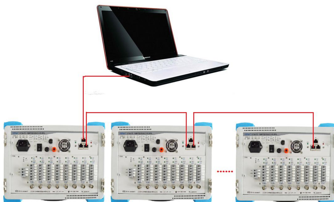
多台仪器逐级扩展连接图
