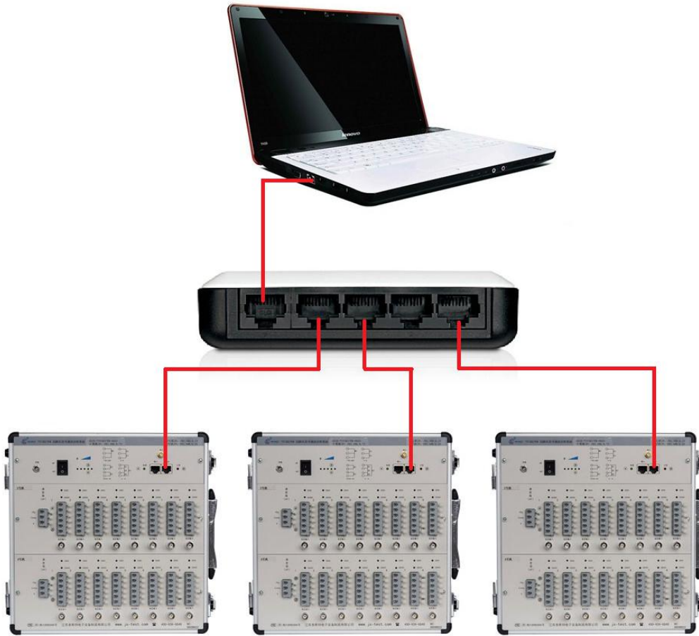
多台仪器网络 HUB 扩展连接图
